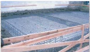
●基礎 (地中梁)
